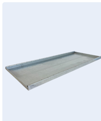
Varenr. 431V0105-100 Galvaniseret hylde for KS-1 og KS-0.5 forberedt for skilleplader Udv. mål i mm.: H:30 B:995 D:405
