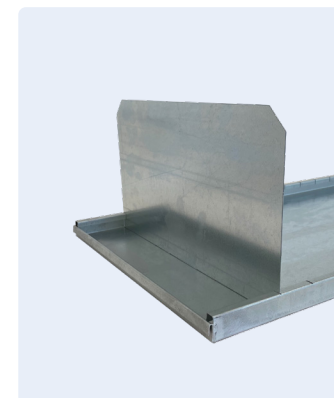
Varenr. 430E0020-100 Galvaniseret skilleplade (stor) for KS-1 og KS-0.5 hylde Udv. mål i mm.: H:230 B:1,25 D:400
