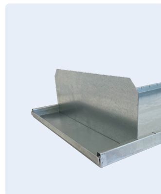
Varenr. 430E0030-100 Galvaniseret skilleplade (lille) for KS-1 og KS-0.5 hylde Udv. mål i mm.: H:150 B:1,25 D:400
